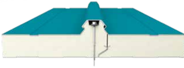
Birleşim Detayı / Connection Detail
