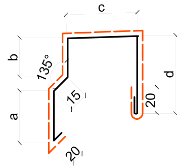
Harpuşta Profili / Eaves Gutter Parapet Profile
