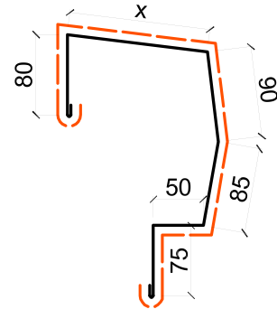
Harpuşta Profili / Eaves Gutter Parapet Profile
