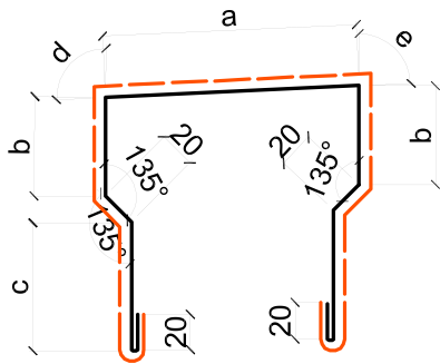
Harpuşta Profili / Eaves Gutter Parapet Profile
