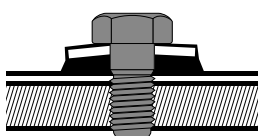
Doğru Vidalama
