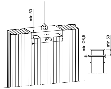
Şekil 9 A - Dikey Kaldırma / Vertical Lift
